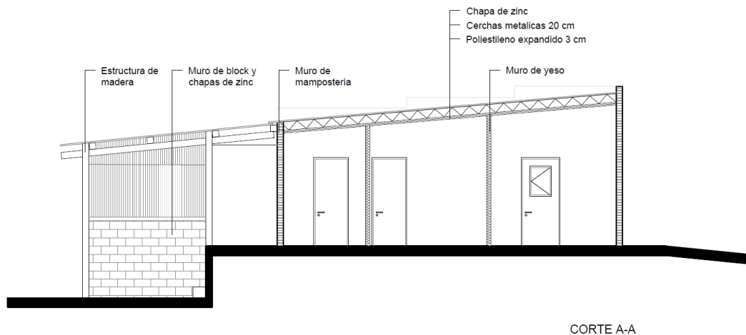
Imagen 3.5 – Corte longitudinal
