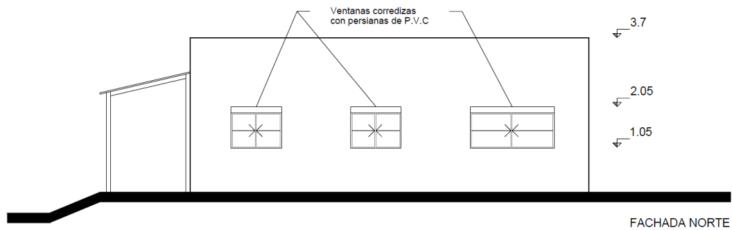
Imagen 3.4 – Fachada norte
