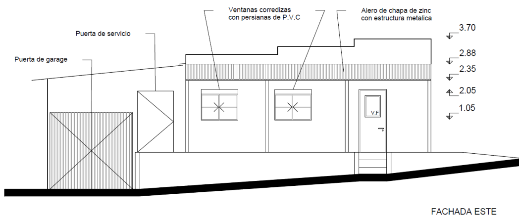
Imagen 3.3 – Fachada este
