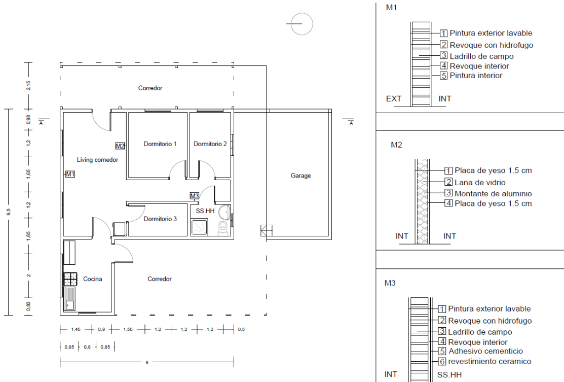
Imagen 3.2 – Planta
